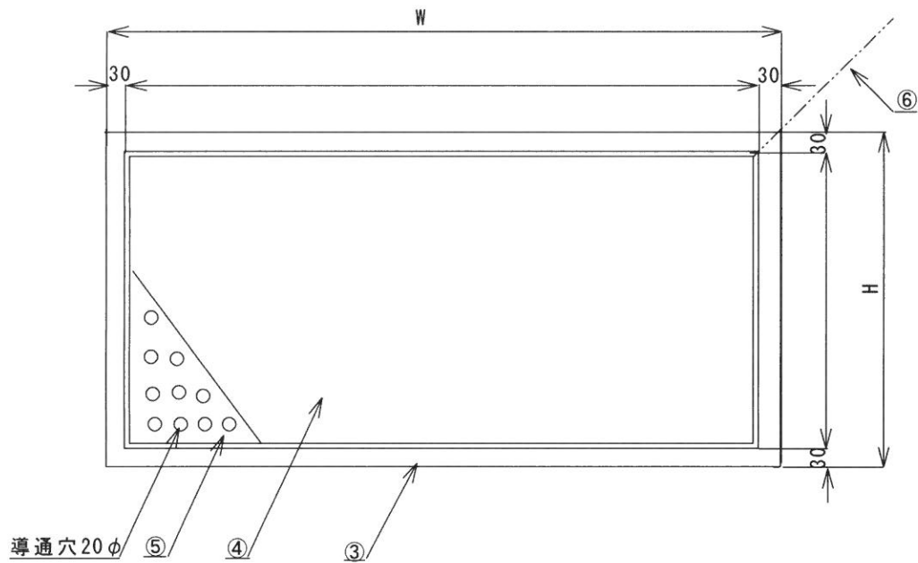
展開図
