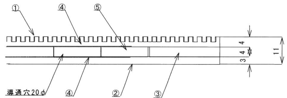
A-A断面図 (1/1)
