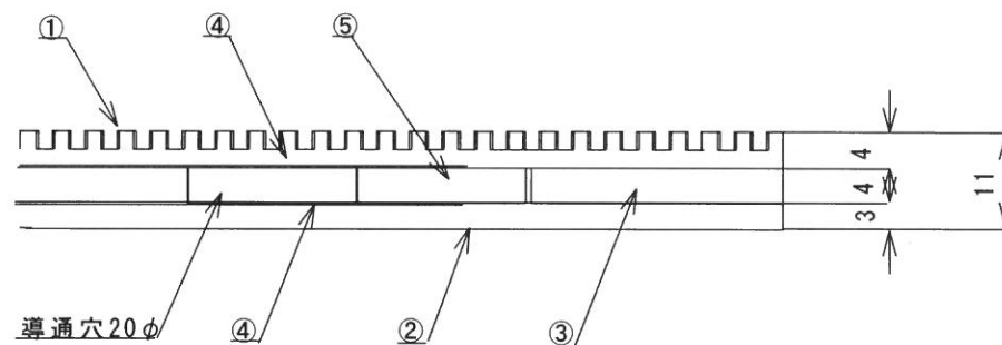
A-A断面図 (1/1)
