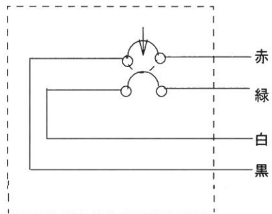
内部結線図
