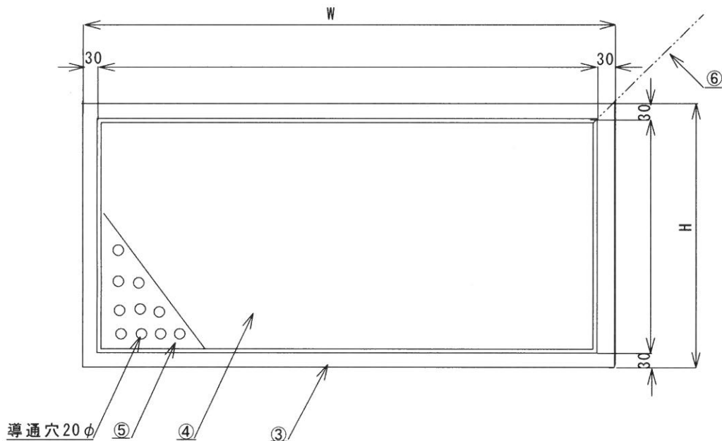
展開図
