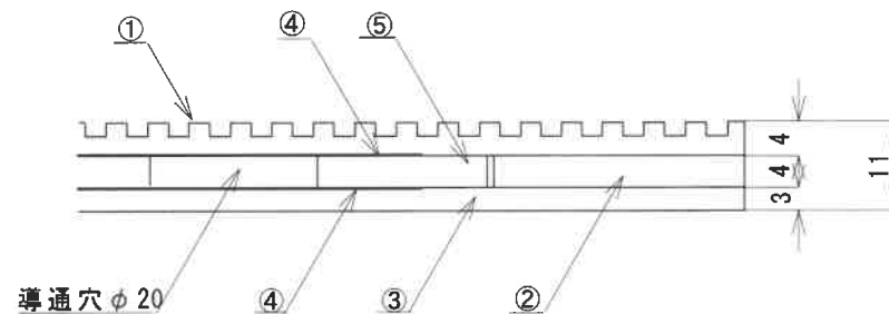
A-A'断面図
