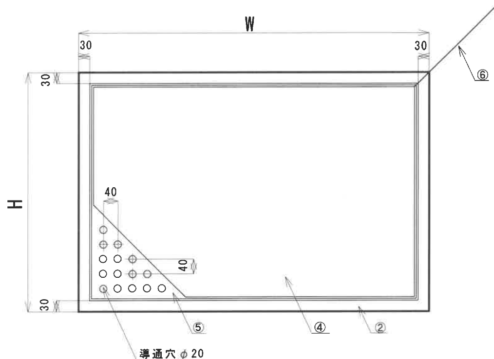
展開図
