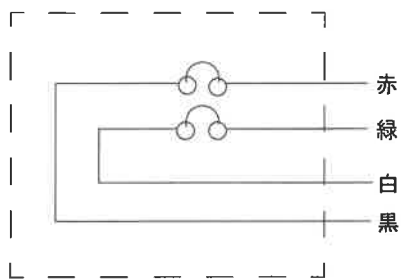
内部結線図
