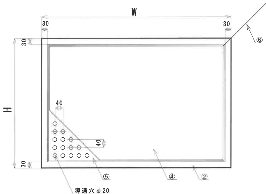
展開図
