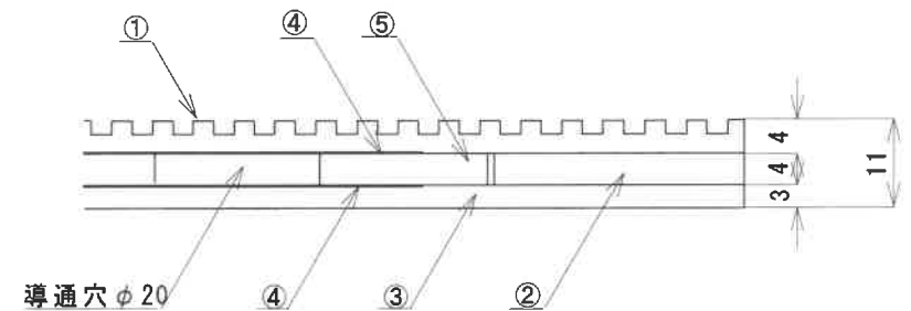
A-A'断面図
