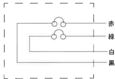
内部結線図
