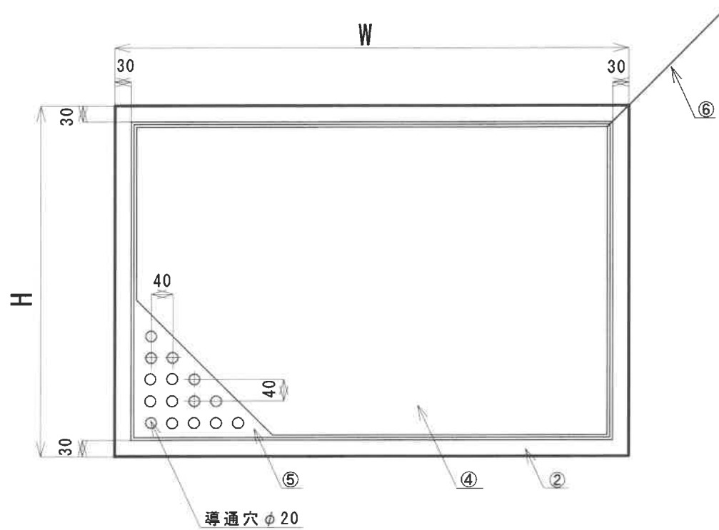
展開図
